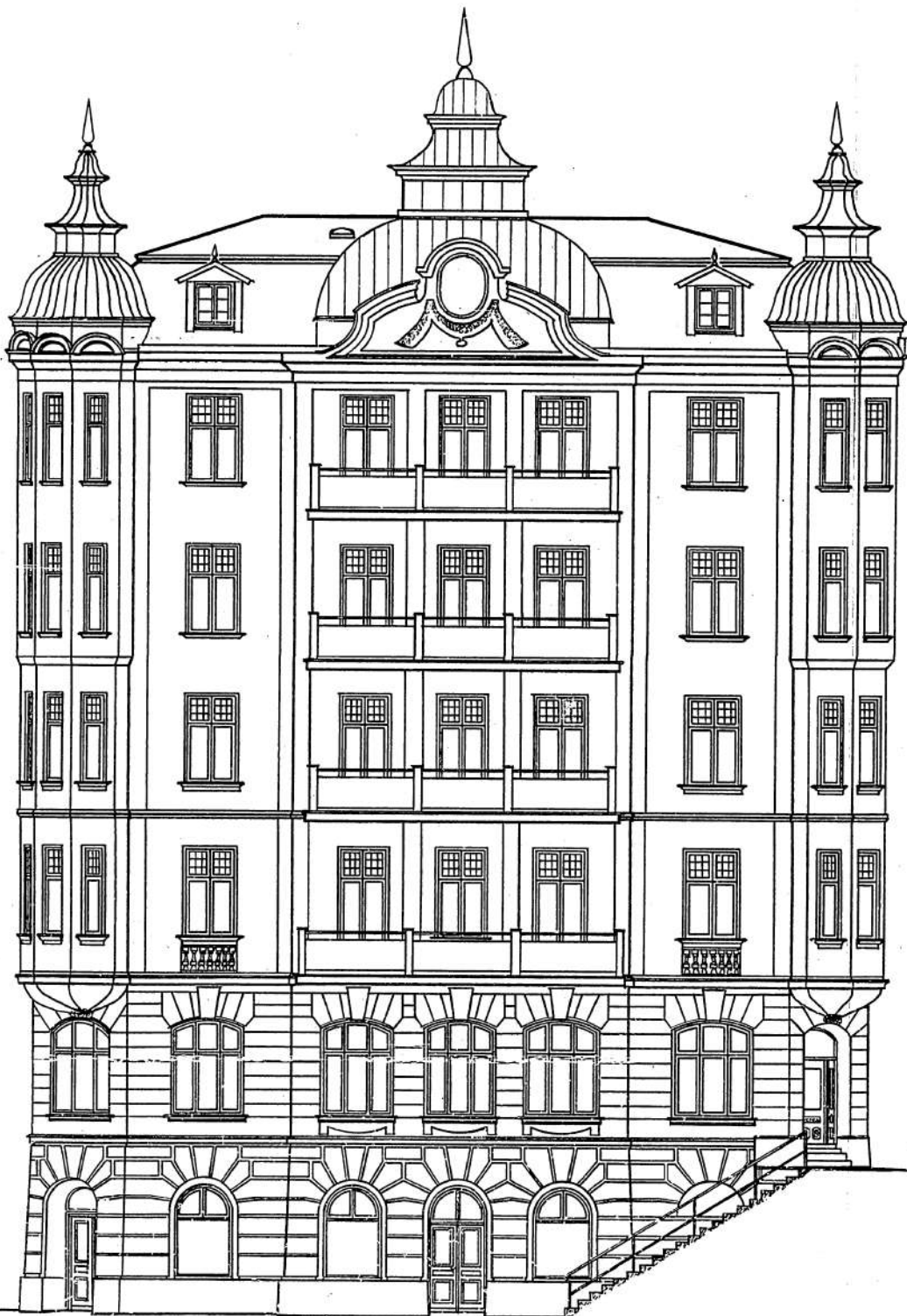
FASAD MOT SÖDER, 1:100
